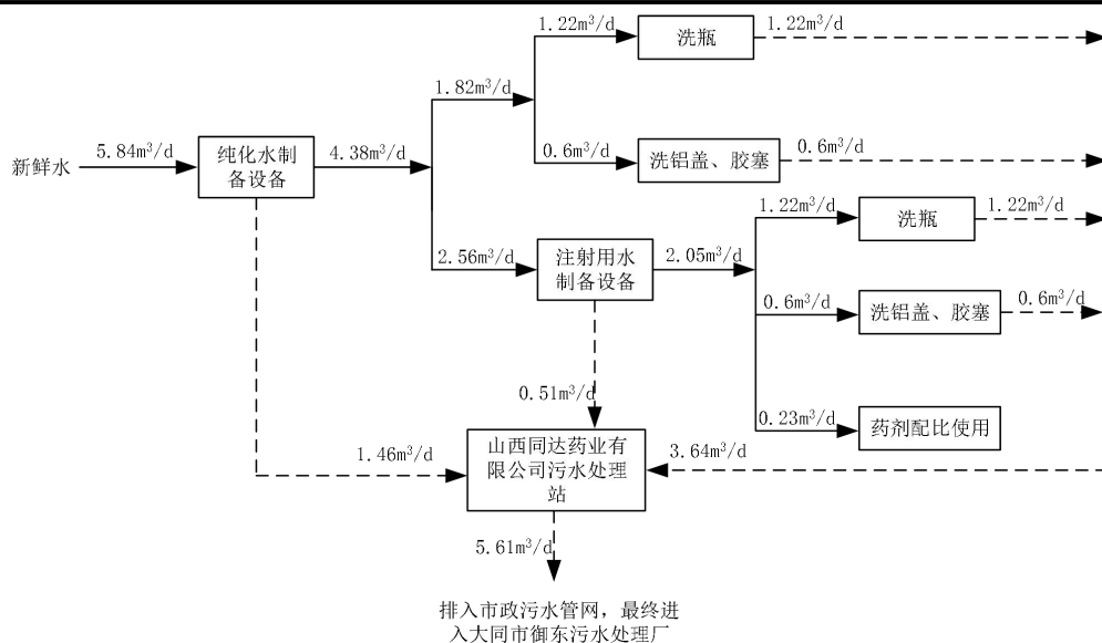
图 2.7-1 本项目水平衡图（单位：m³/d）
