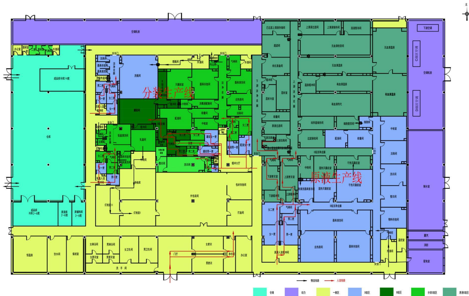
附图3-1 生物制剂车间总平面布置图
