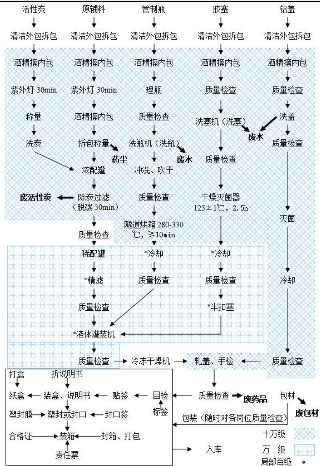
图 2.14-2 粉针剂生产工艺流程图及产污环节
