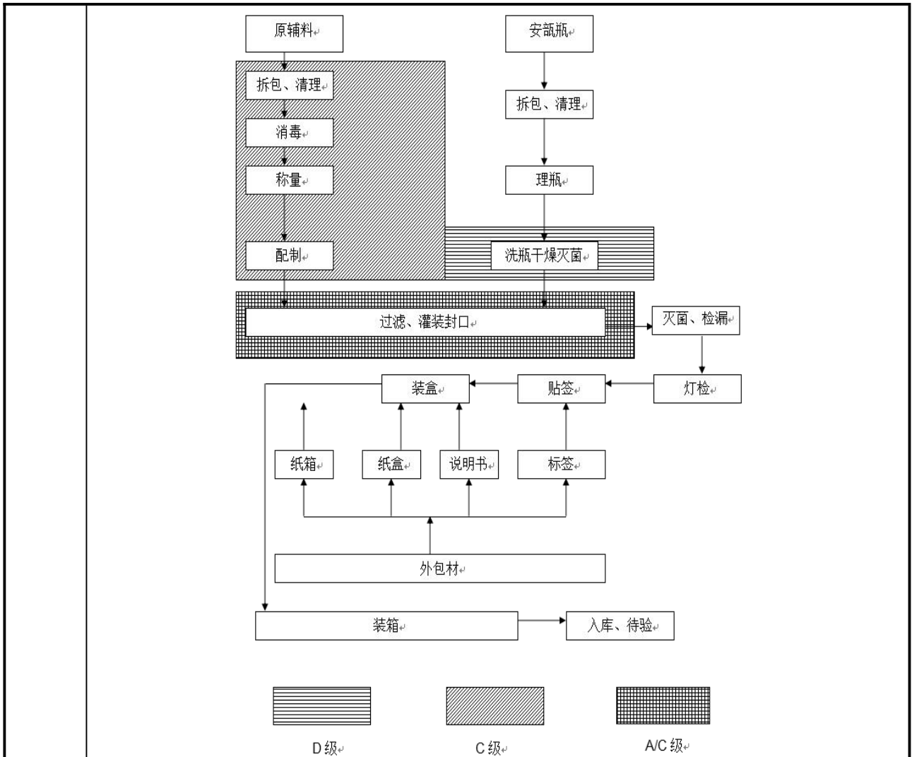
图 2.14-2 水针剂生产工艺流程图及产污环节
