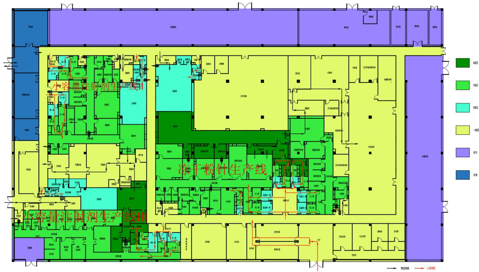
附图3-2 冻干粉针车间总平面布置图
