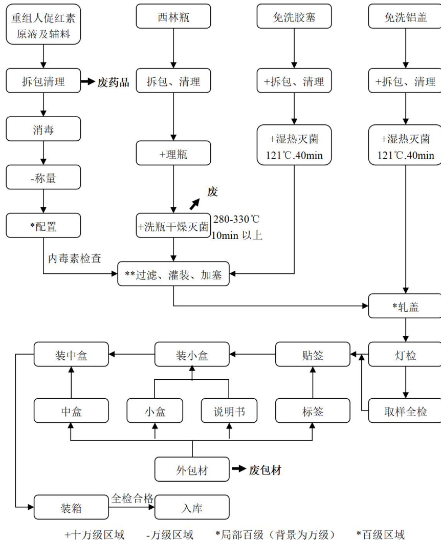
图 2.14-1 人促红素注射液生产流程图及产污环节
